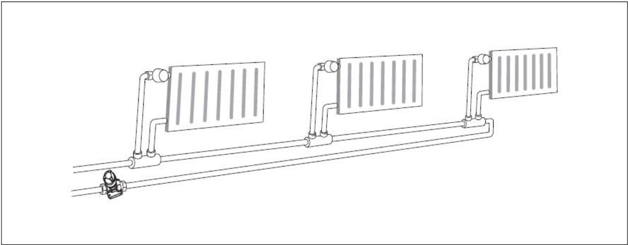
Рис. 6. Пример применения клапанов балансировочных автоматических комбинированных типа АВ-QM на стояках однотрубной системы отопления.
