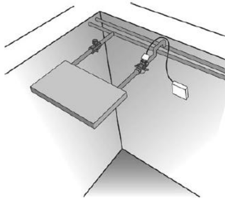
Рис. 4. Пример применения клапанов балансировочных автоматических комбинированных типа АВ-QM на обвязке охлаждающих потолочных панелей в системах с переменными гидравлическими характеристиками.
