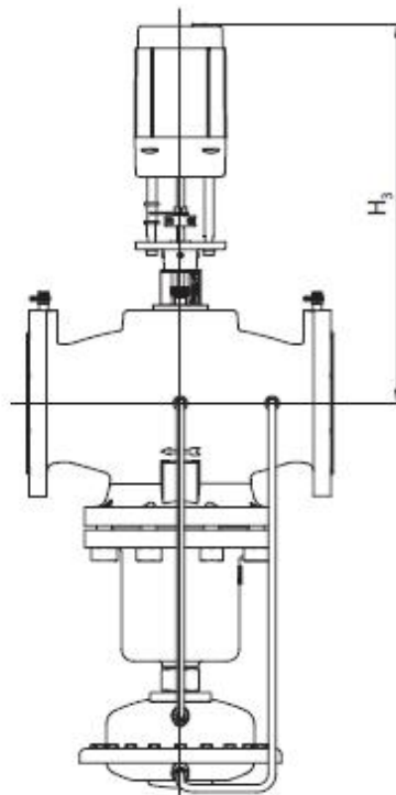
AME 55 QM + AV-QM D_y = 125 мм
