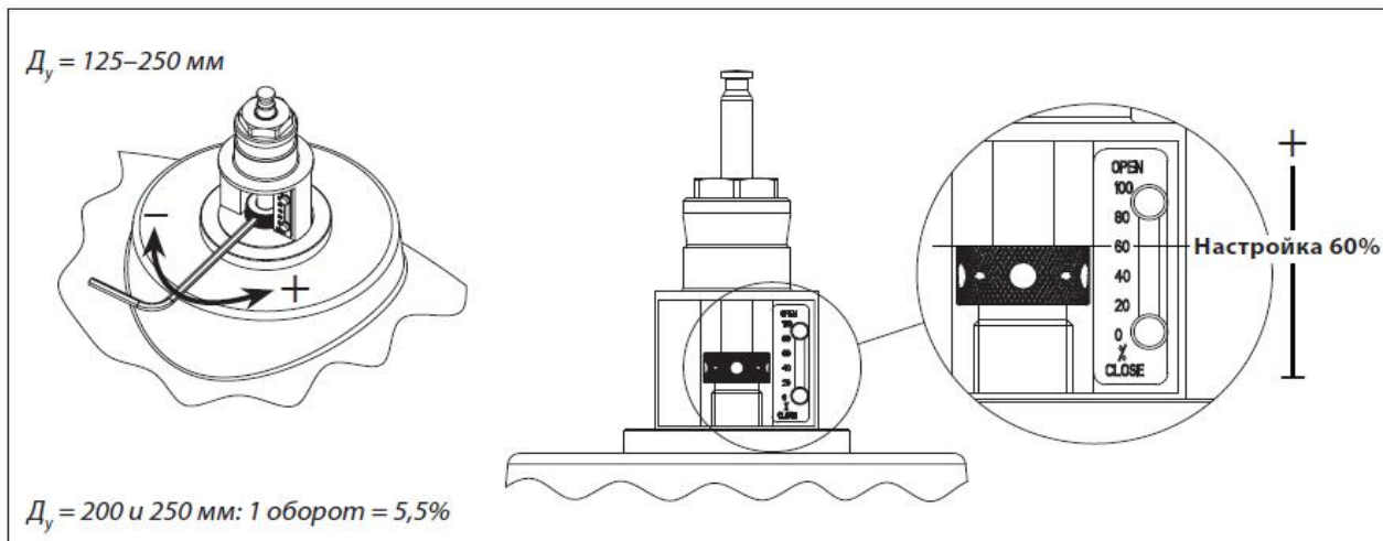
Рис.14. Пример настройки клапана типа АВ-QM D_y = 125 - 250 мм
