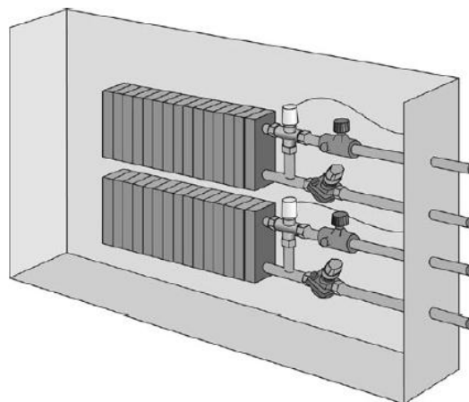
Рис. 5. Пример применения клапанов балансировочных автоматических комбинированных типа АВ-QM на обвязке фэнкойлов в системах с постоянными гидравлическими характеристиками.
