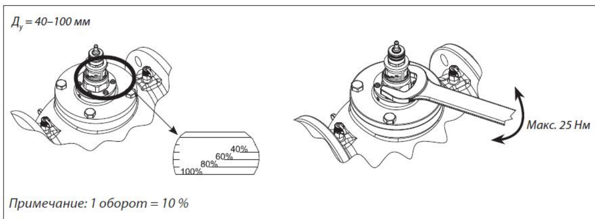
Рис.13. Пример настройки клапана типа АВ-QM D_y = 40 - 100 мм
