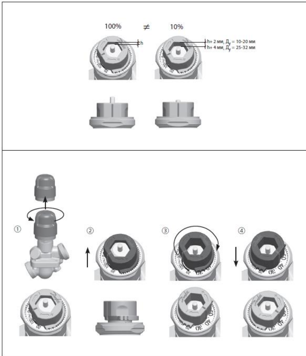
Рис.12. Пример настройки клапана типа АВ-QM D_y = 10 - 32 мм
